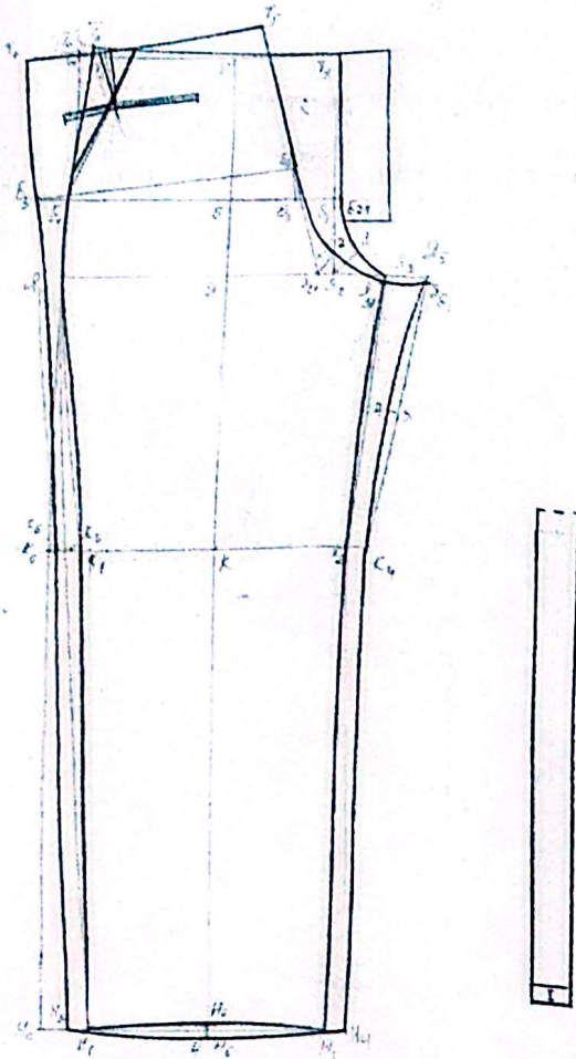
2-сурет. Шалбардың сызбасы
